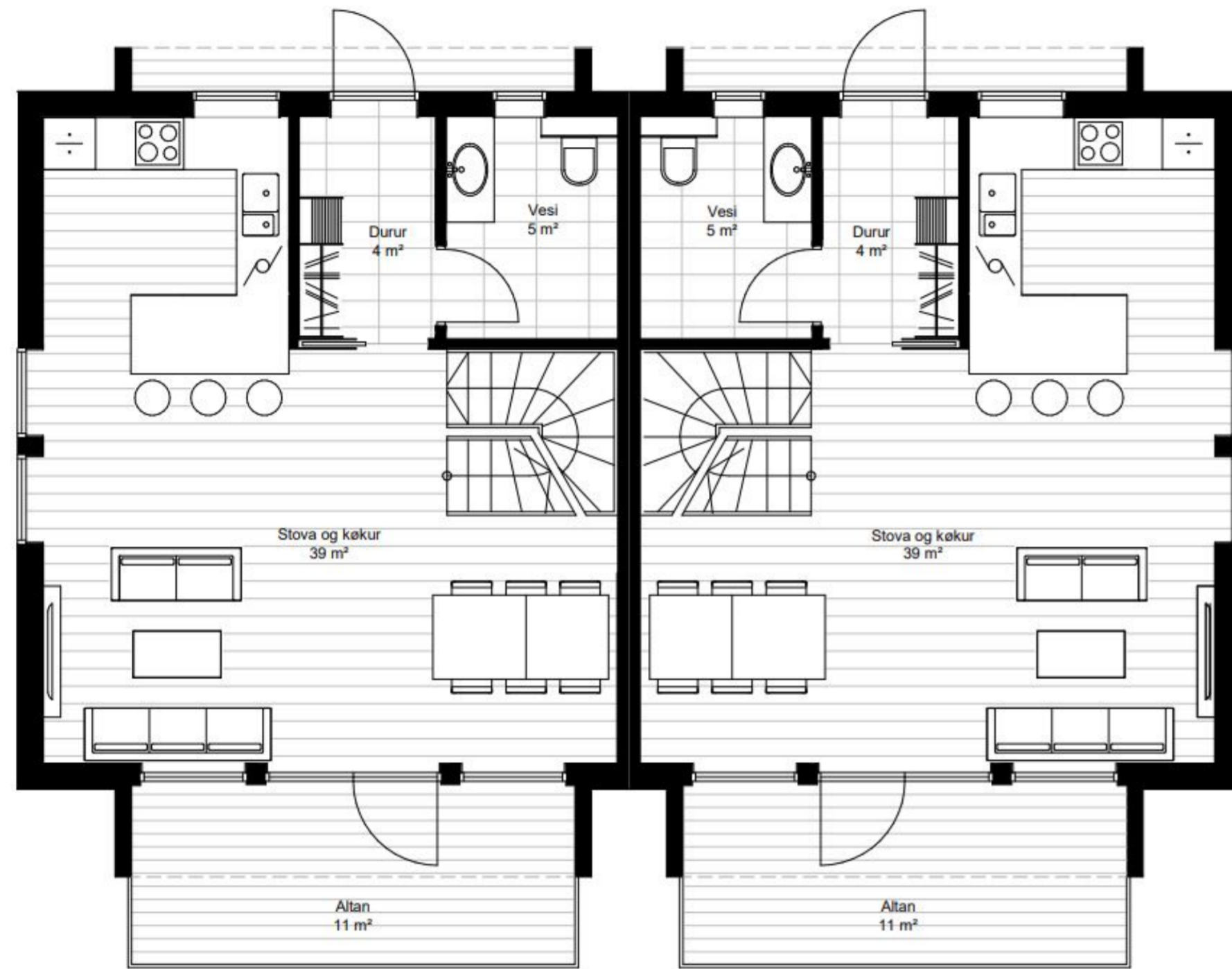
Flatmynd 1. hædd
