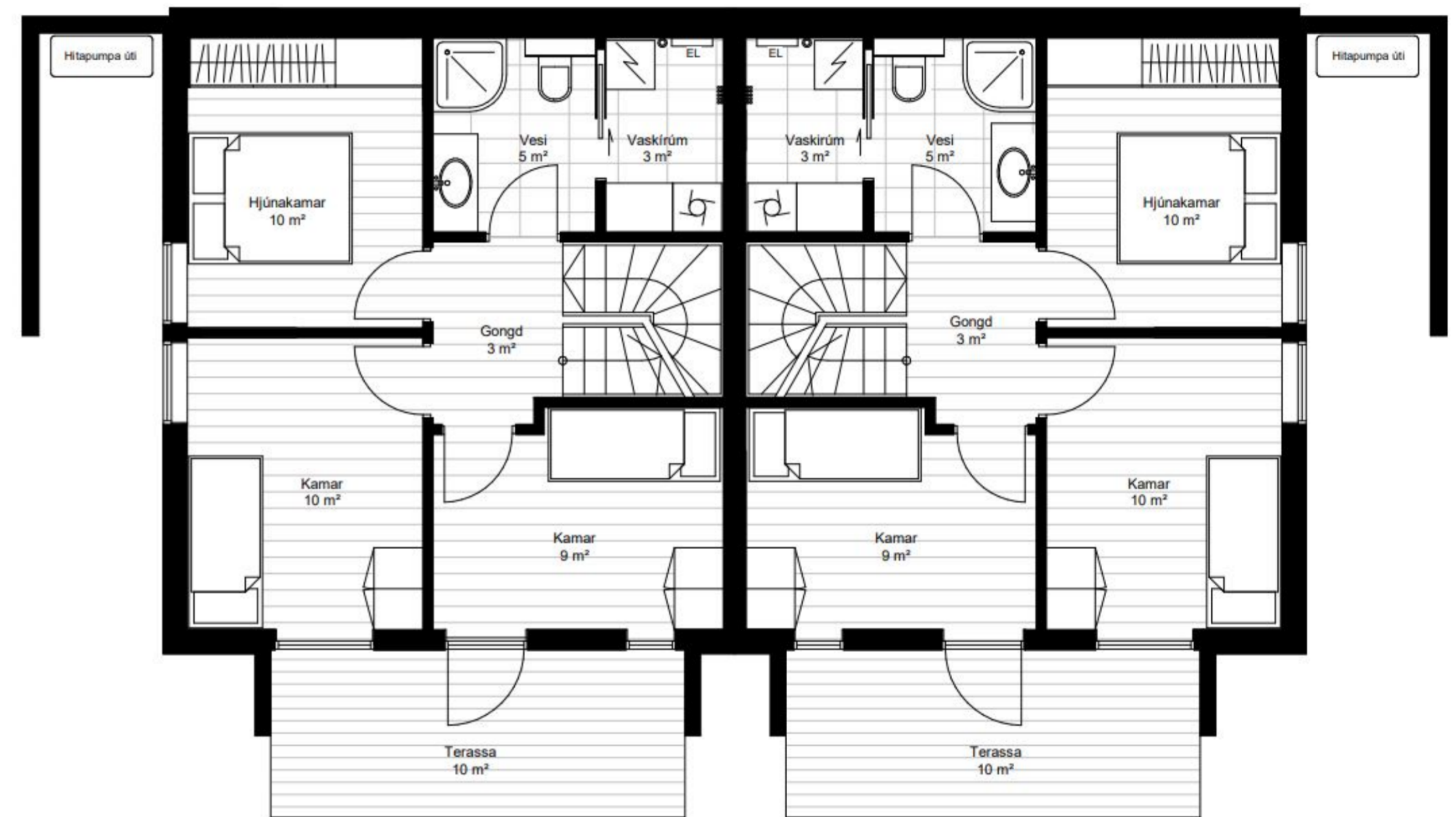
Flatmynd kjallari
